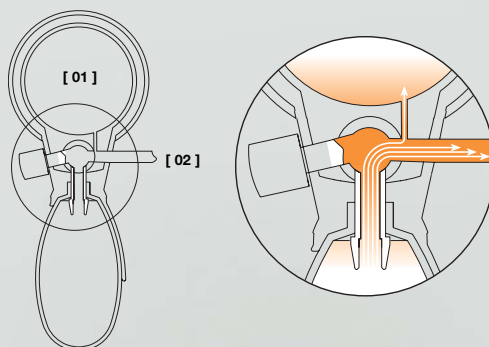
[ 01 ] MANOMETRO [ 02 ] RACCORDO PER BRACCIALE
